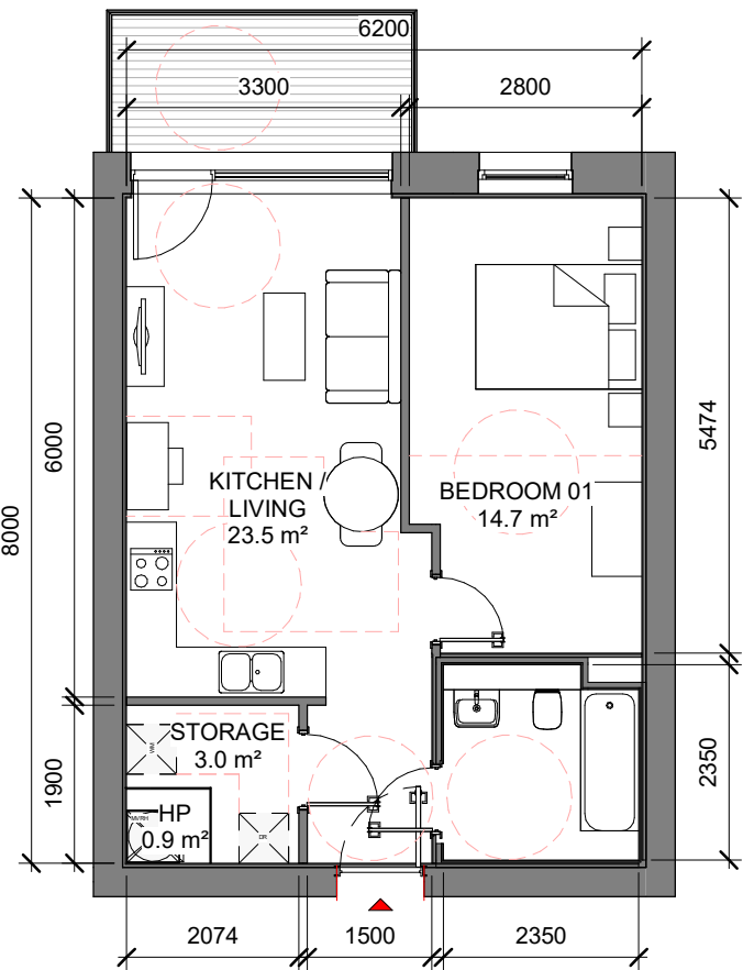
1 1B_2P_07 UD 1 : 100
