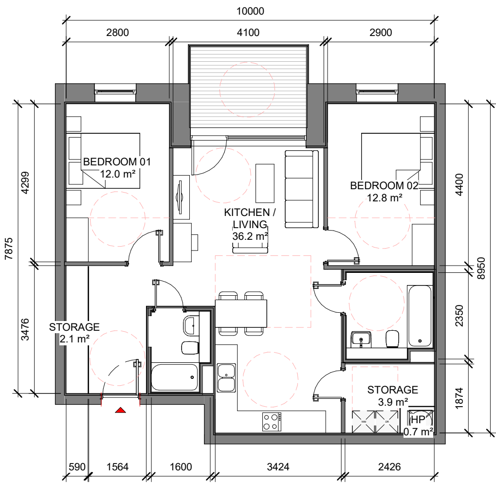
2 2B_4P_07 UD 1 : 100
