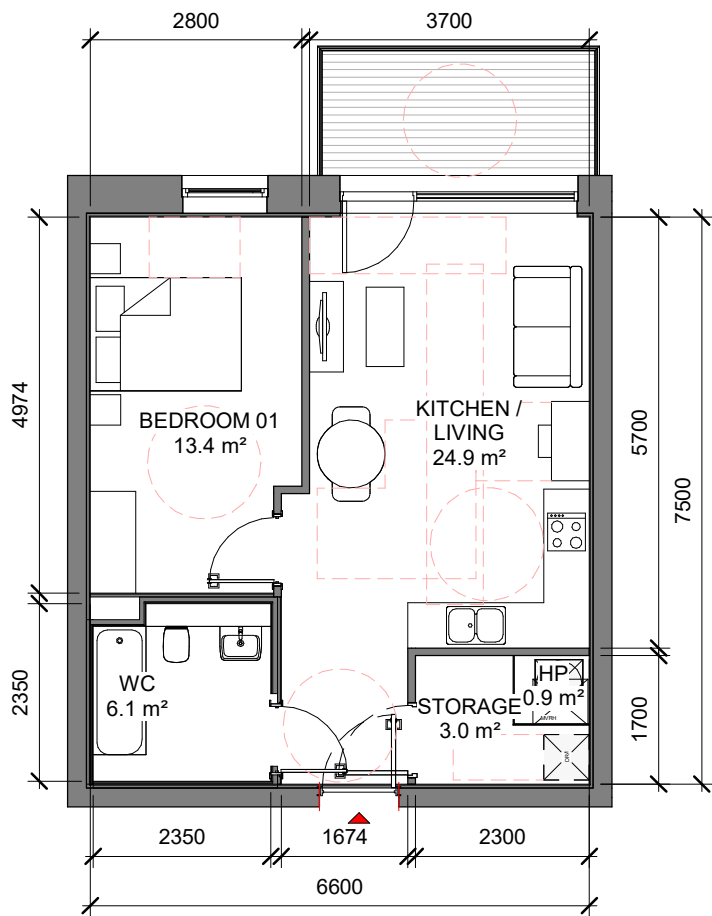
3 1B_2P_01 UD 1 : 100
