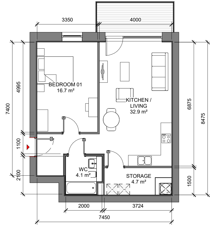
4 1B_2P_04 1 : 100
