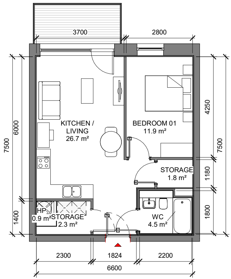
1 1B_2P_01 1 : 100
