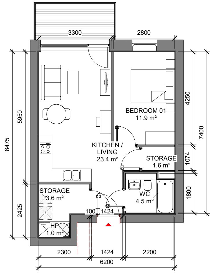
3 1B_2P_03 1 : 100
