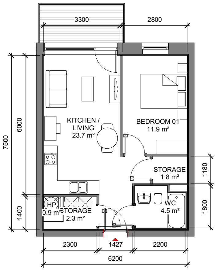
2 1B_2P_02 1 : 100
