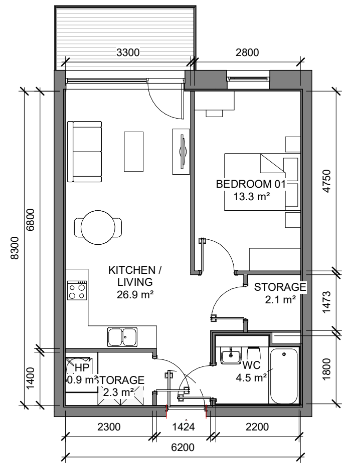
5 1B_2P_05 1 : 100
