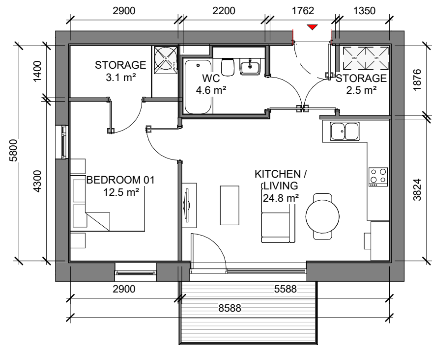
8 1B_2P_08 1 : 100
