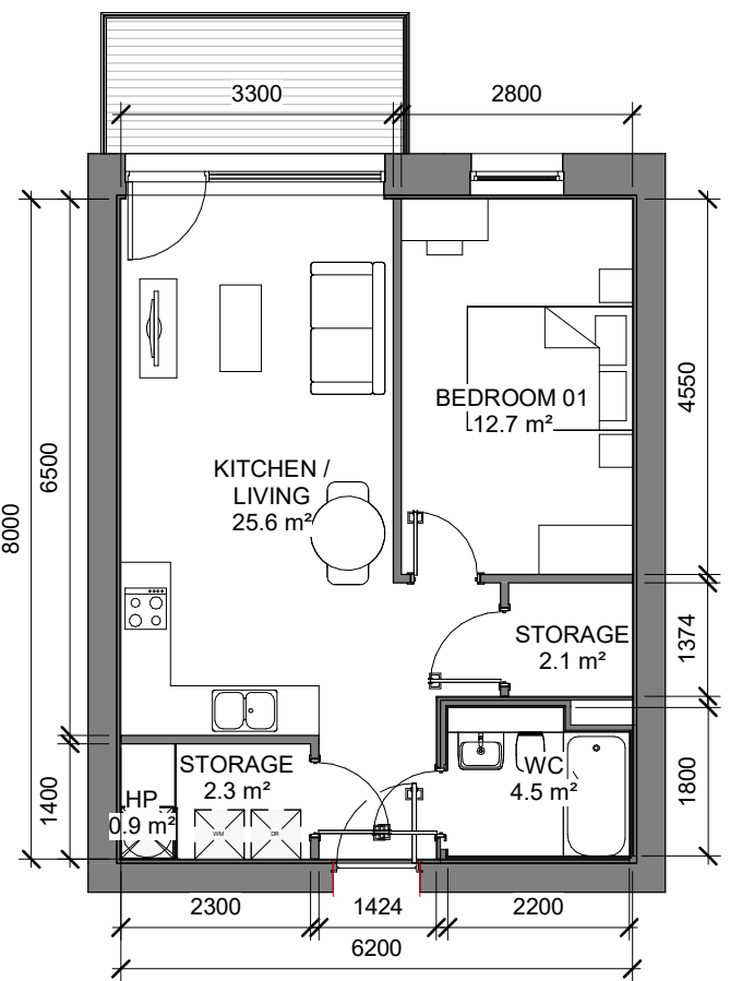
7 1B_2P_07 1 : 100
