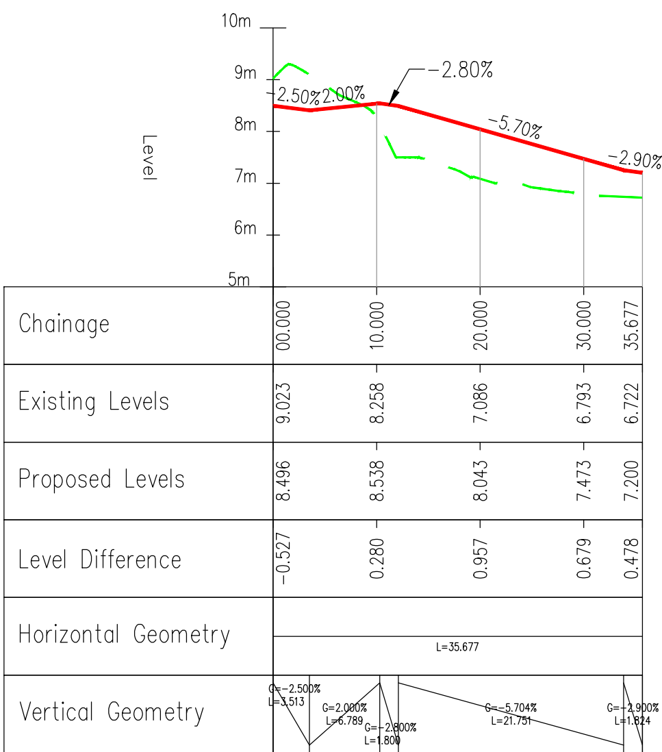
RAMP – LONGSECTION SCALE: H 1:500,V 1:100. DATUM: 5.000
