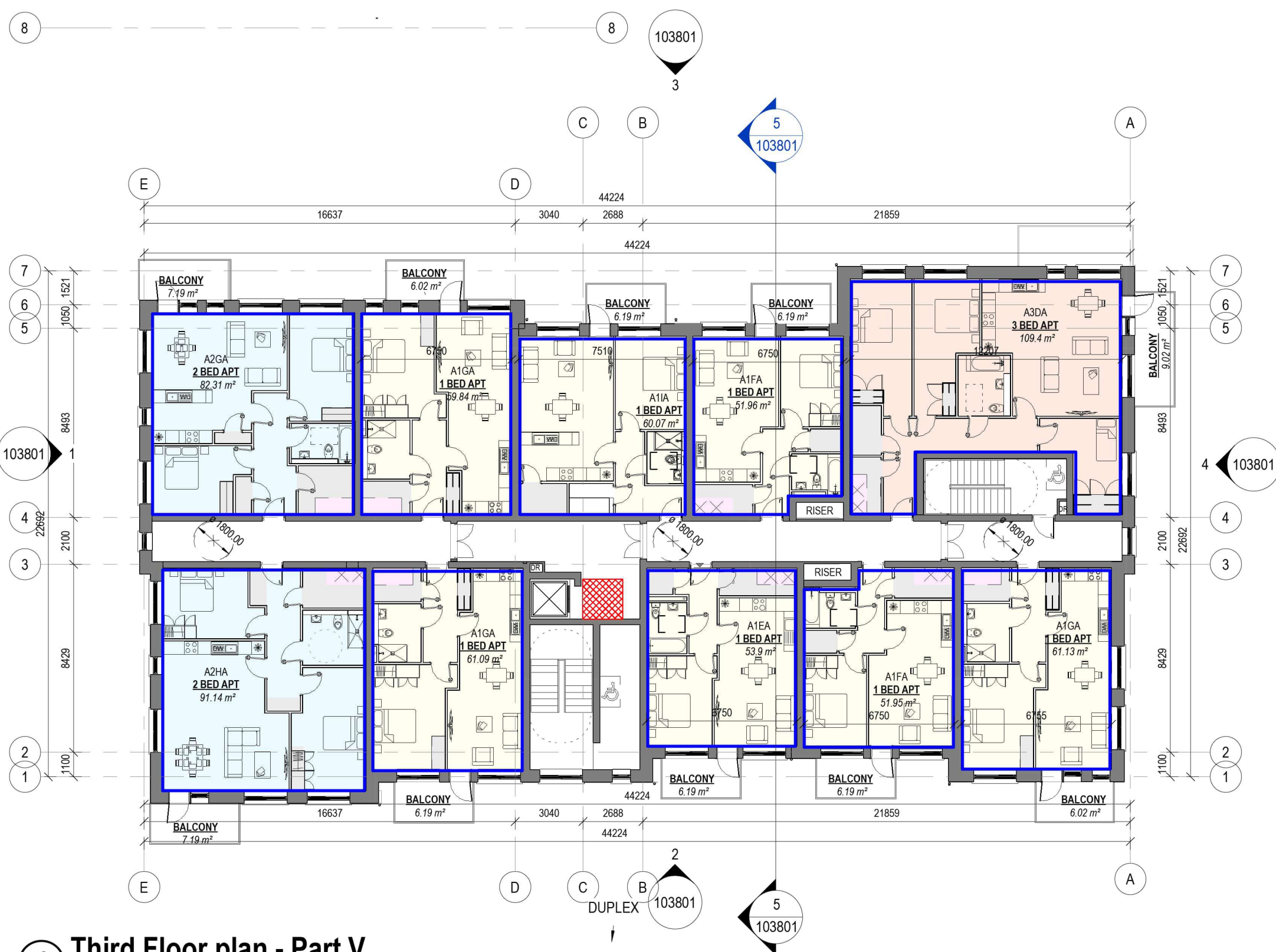
Scale: 1 : 200
