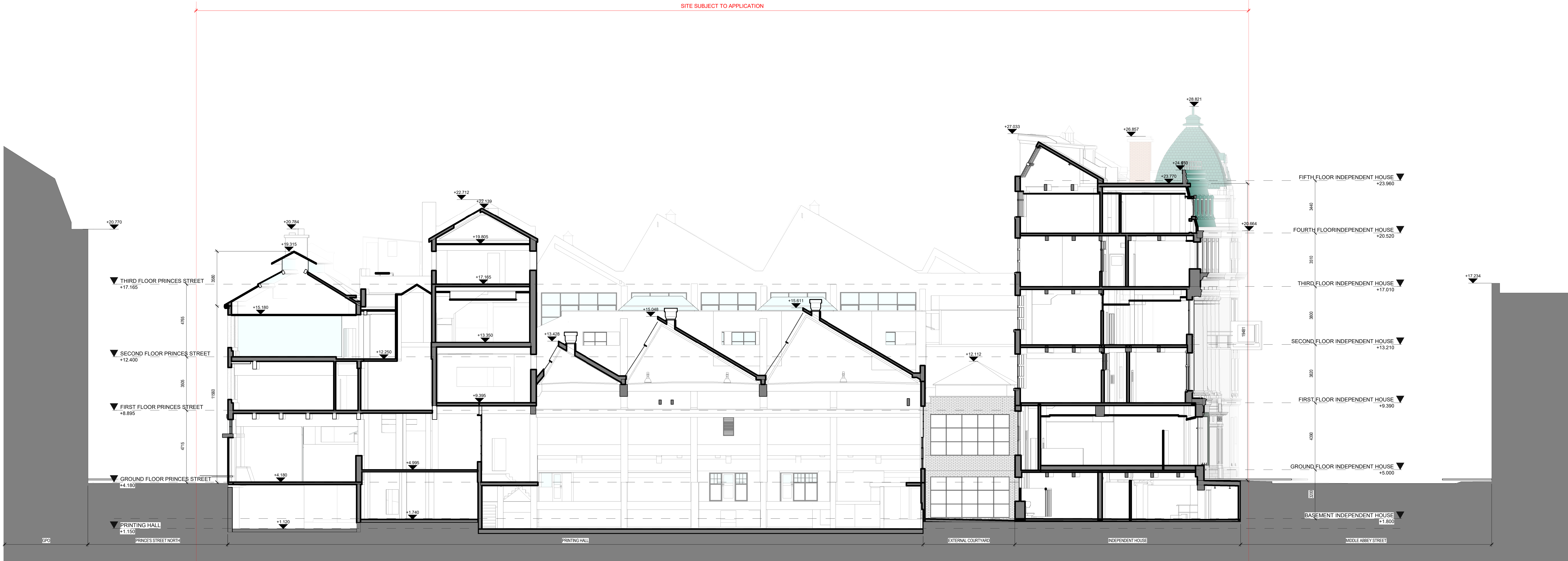
2 SECTION BB EXISTING 1 : 100
