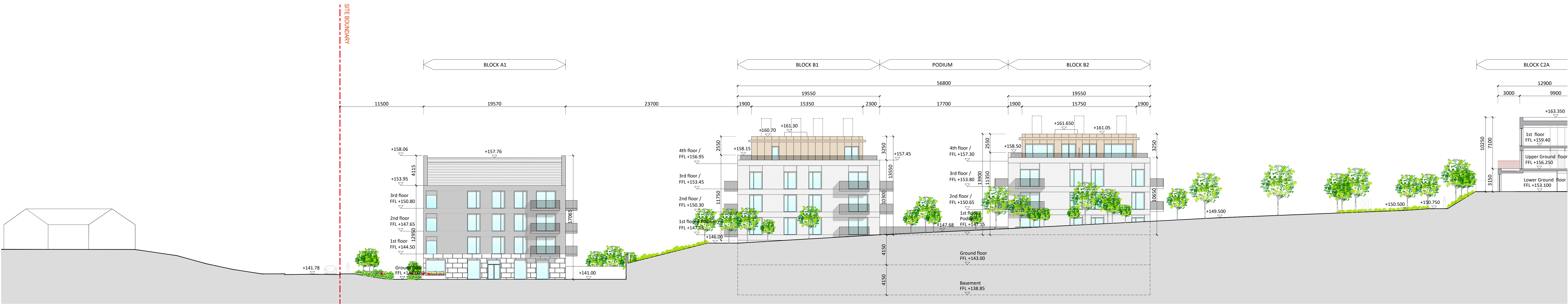
Contiguous site elevation AA. 1/200 @ A0
